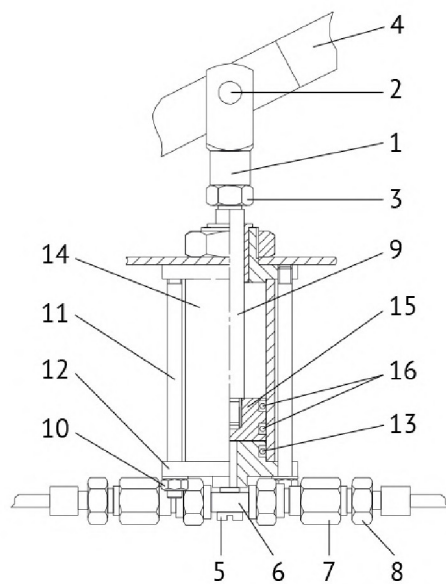
Рис. 3. Устройство насоса:
