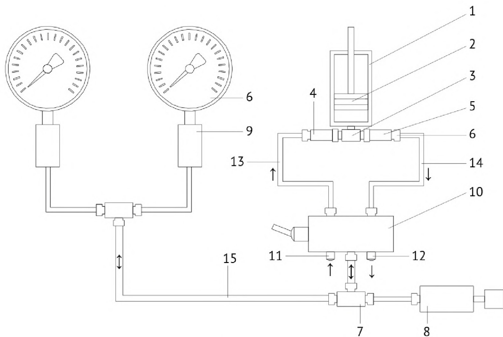
Рис. 2. Пневматическая схема ПУСК:
